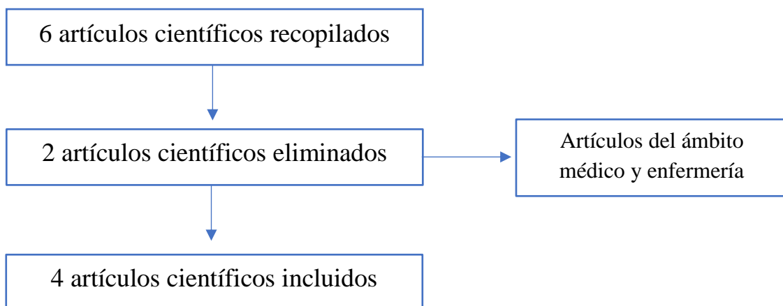
Gráfico 2. Diagrama de Flujo Prisma
