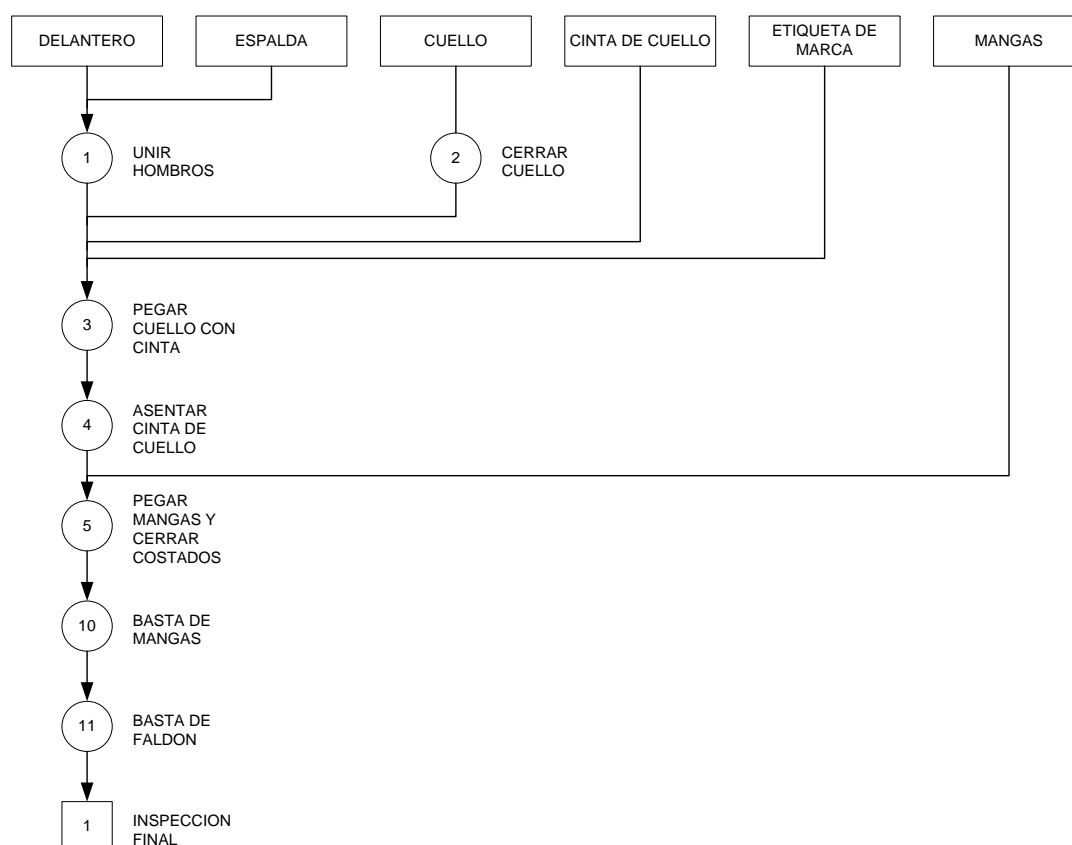
Figura 7 Diagrama de ensamble t-shirt básico
