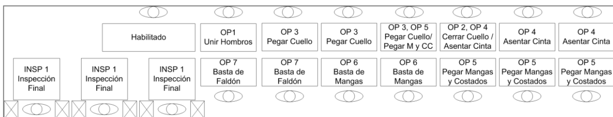
Figura 17 Layout típico de la línea esbelta de costura - t-shirt básico
